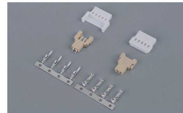
CB2.0(2.0mm)
