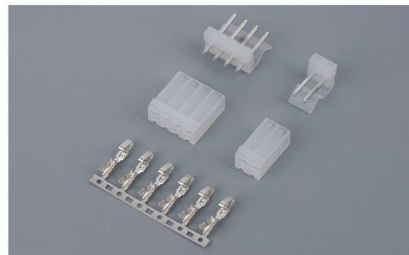
3.96(3.96mm)
