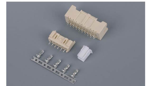
XA(2.5mm)
