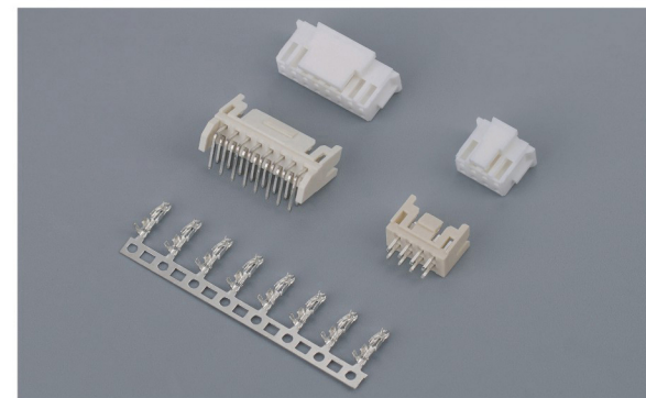
PHC(2.0mm)
