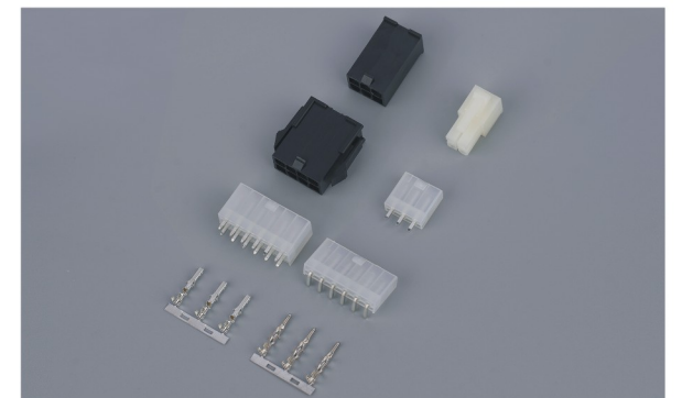
5556-5569(4.2mm)
