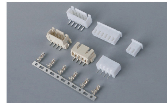
XH(2.5mm)
