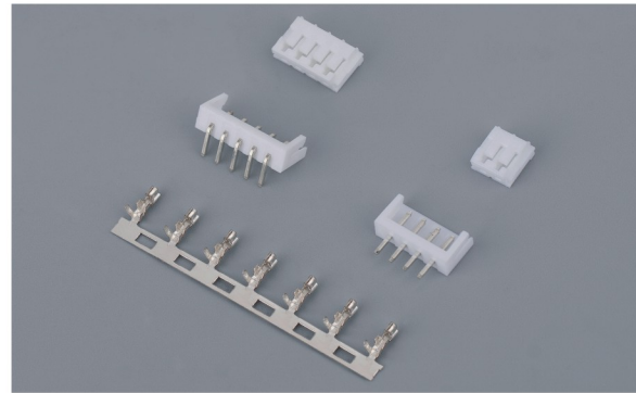
EH(2.5mm)
