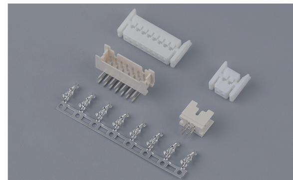
PHDS(2.0mm)
